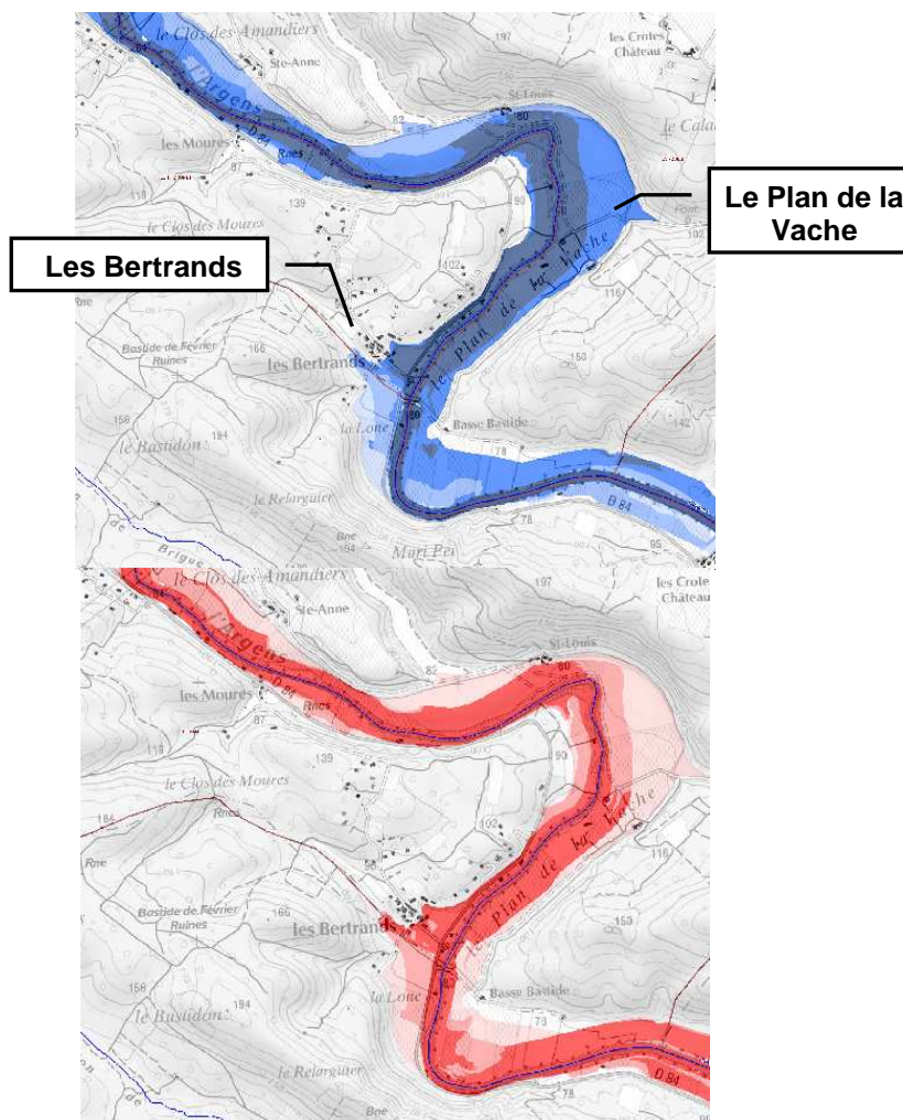
Figure 33: Hauteur d'eau et vitesses d'écoulement – L'Argens à l'aval de la confluence avec le Vallon de Saint Peyre
