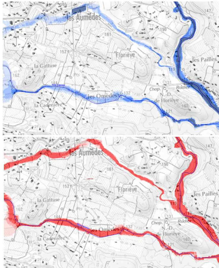
Figure 25: Hauteur d'eau et vitesses d'écoulement – Le Réal Calamar depuis la zone d'activités jusqu'à la confluence avec la Florièye
