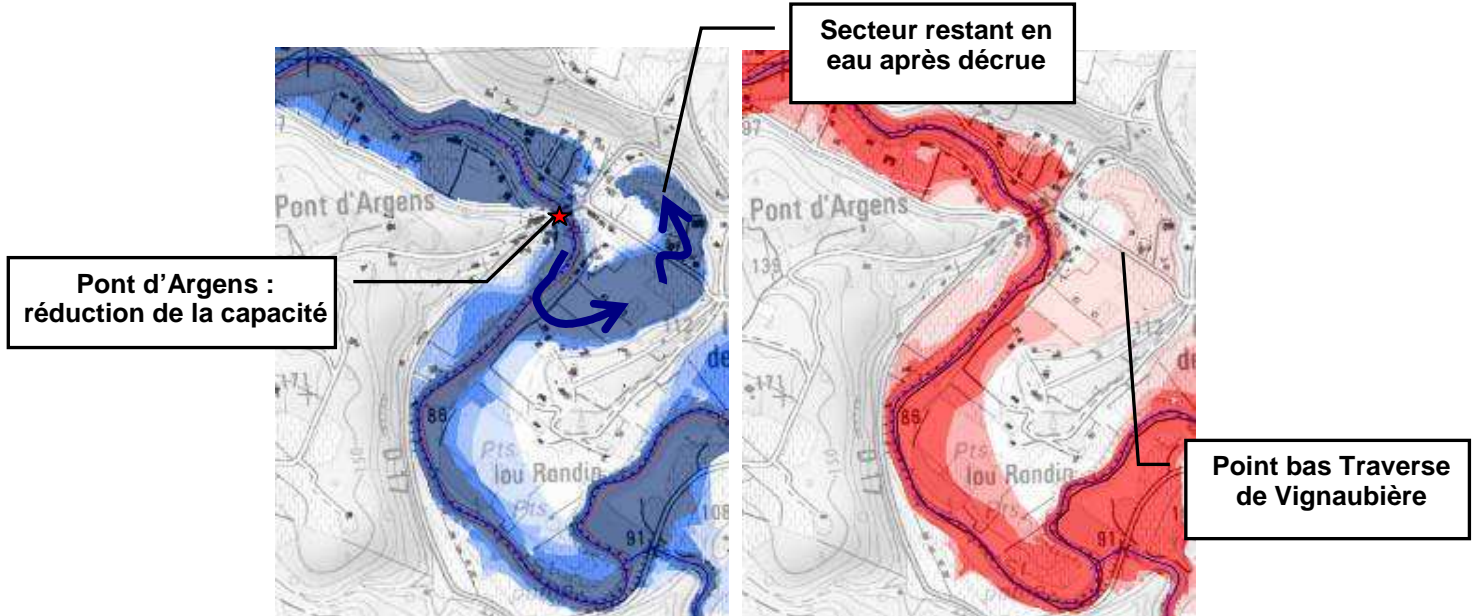
Figure 32: Hauteur d'eau et vitesses d'écoulement - L'Argens au niveau du pont d'Argens
